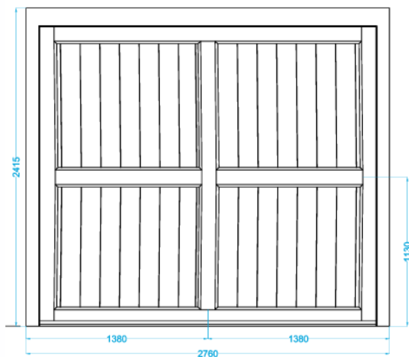
VUE INTERIEURE
