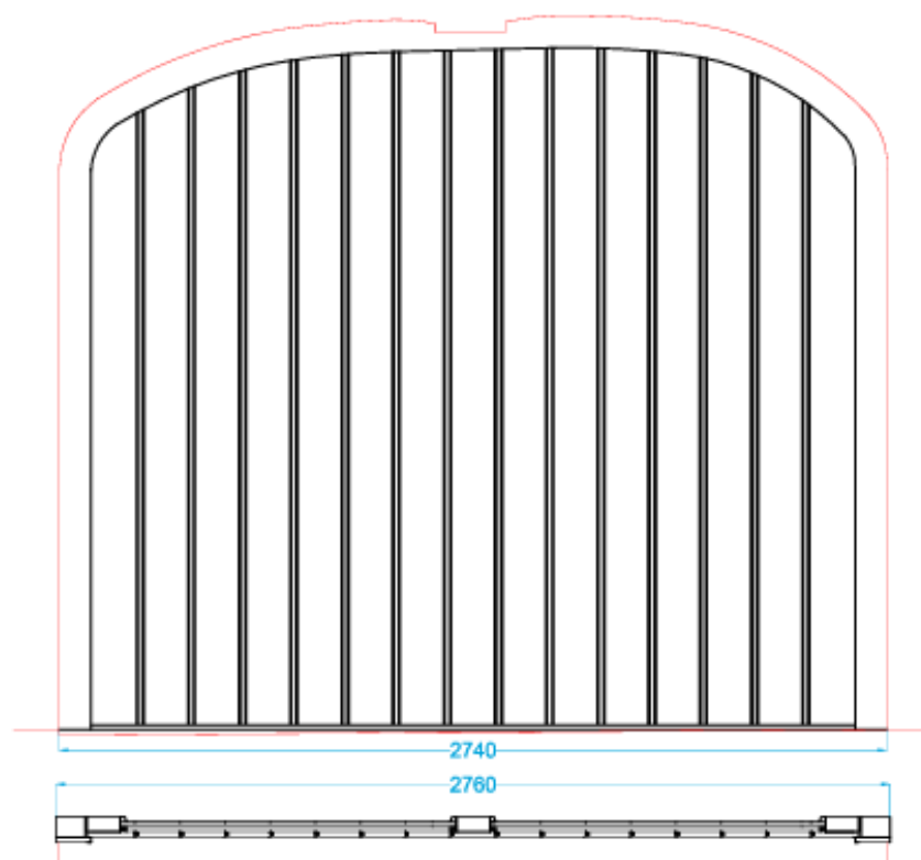
VUE INTERIEURE
